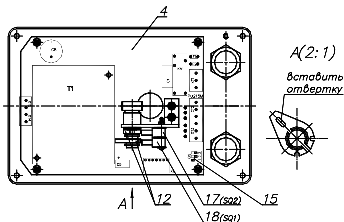
Рисунок 1 - Электропривод ВЭП-115-4000
