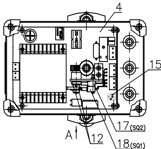
Рисунок 1 - Электропривод ВЭП-115М-4000
