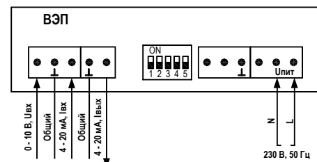
Рисунок 3.1 Схема подключения с управлением аналоговым сигналом.
