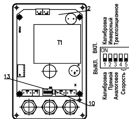
Рисунок 2. ВЭП-135М (вид при снятой крышке)
