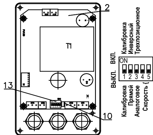
Рисунок 2. ВЭП-138М (вид при снятой крышке)
