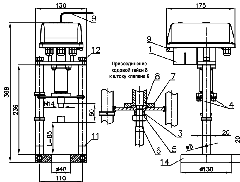
Рисунок 1 - ВЭП-138М
