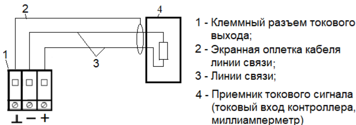
Рисунок Д.2 Схема подключения активного токового выхода расходомера к измерителю тока (без передачи данных по HART)
