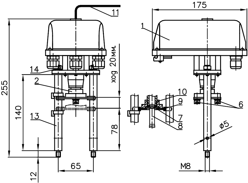
Рисунок 1 - ВЭП-125М
