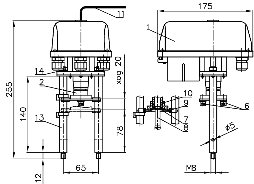
Рисунок 1 - ВЭП-125МВ
