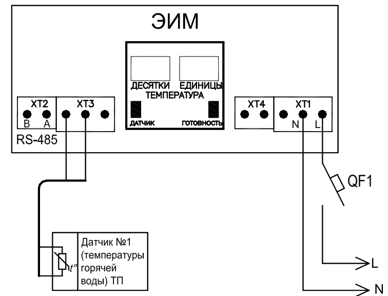
Рисунок 2 - Схема подключения ЭИМ ВЭП-125МВ
