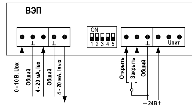
Рисунок 3. Схема подключения.
