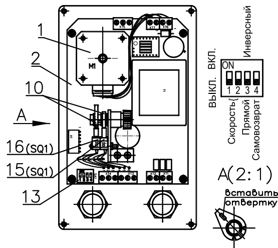
Рисунок 2 - ВЭП-111В (вид при снятой крышке)
