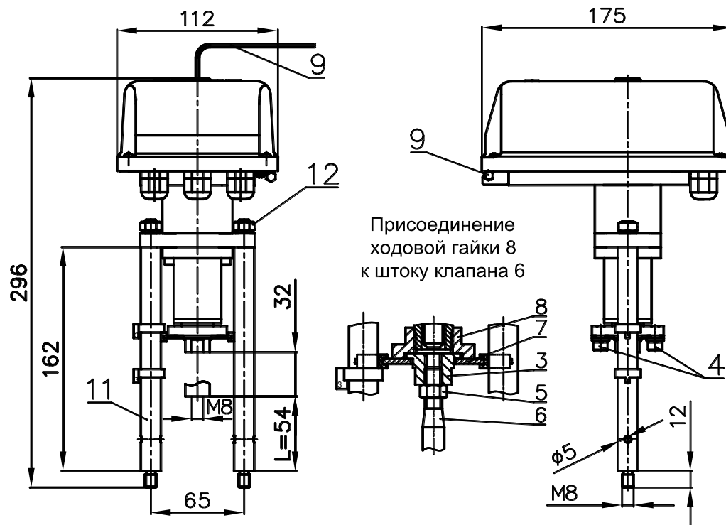
Рисунок 1 - Электропривод ВЭП-115М-3000
