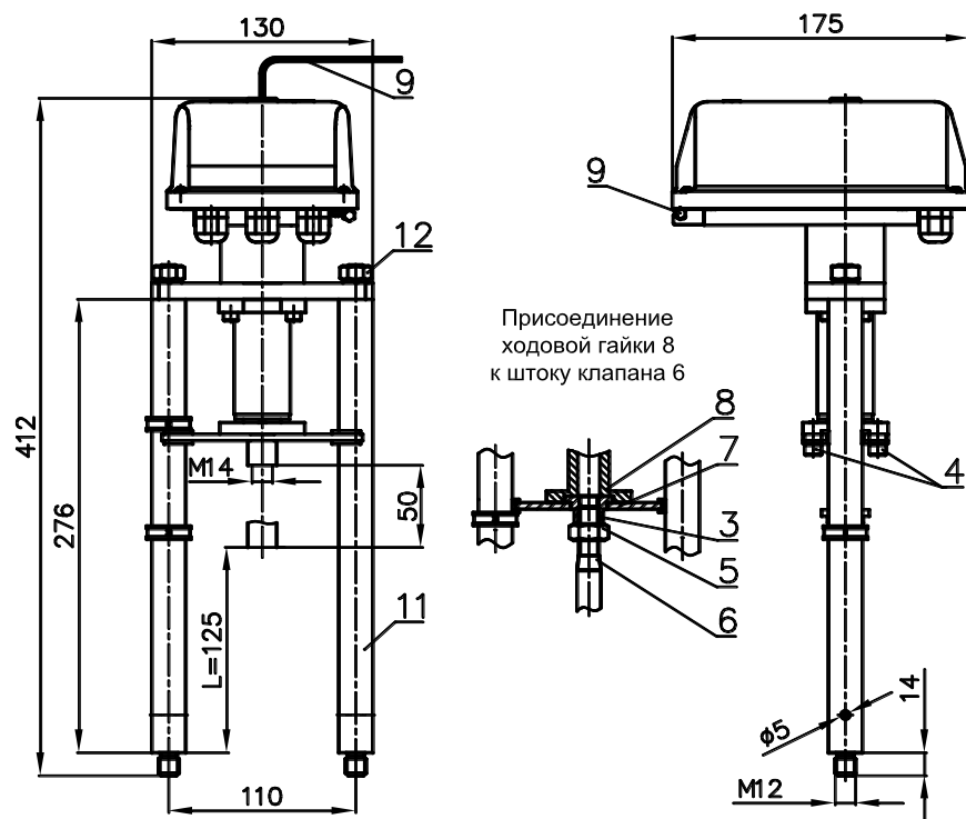
Рисунок 1 - Электропривод ВЭП-115М-4000
