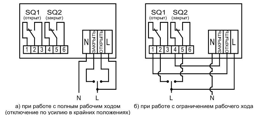
Рисунок - 3 Схема подключения
