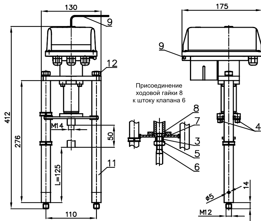
Рисунок 1 - ВЭП-115В
