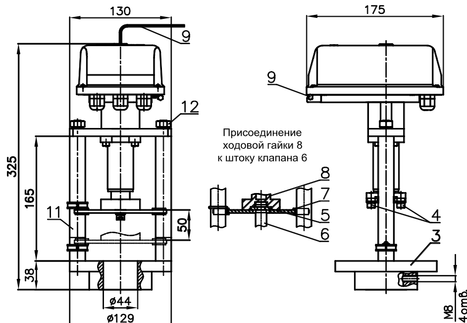
Рисунок 1 - Электропривод ВЭП-118М-01А
