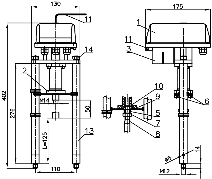
Рисунок 1 - ВЭП-121М
