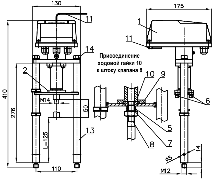
Рисунок 1 - ВЭП-125М
