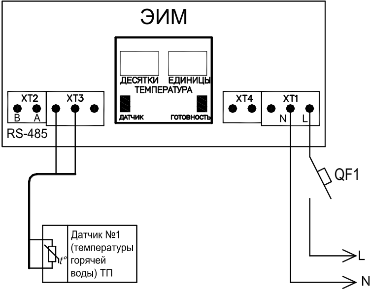
Рисунок 2 - Схема подключения ЭИМ ВЭП-125М 5 СВИДЕТЕЛЬСТВО О ПРИЕМКЕ
