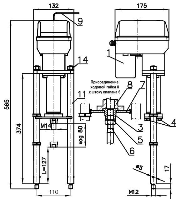
Рисунок 1 - ВЭП-131М
