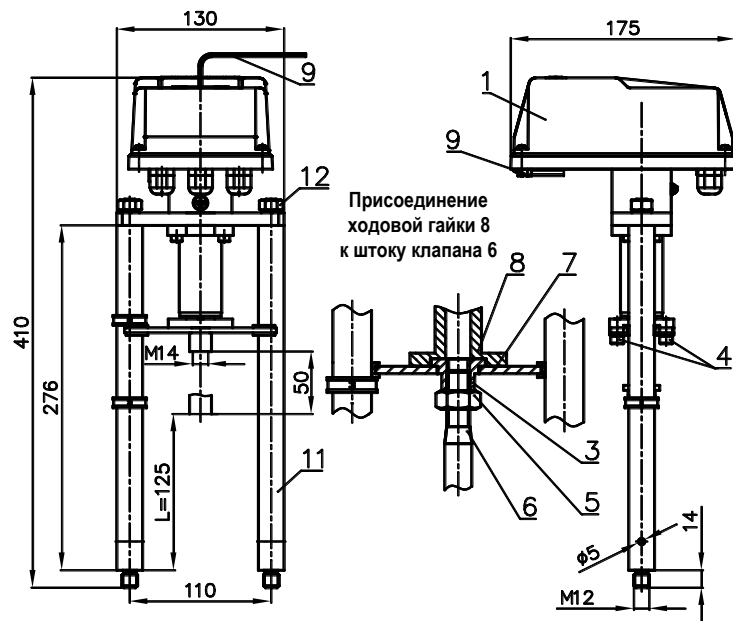
Рисунок 1 - ВЭП-131М
