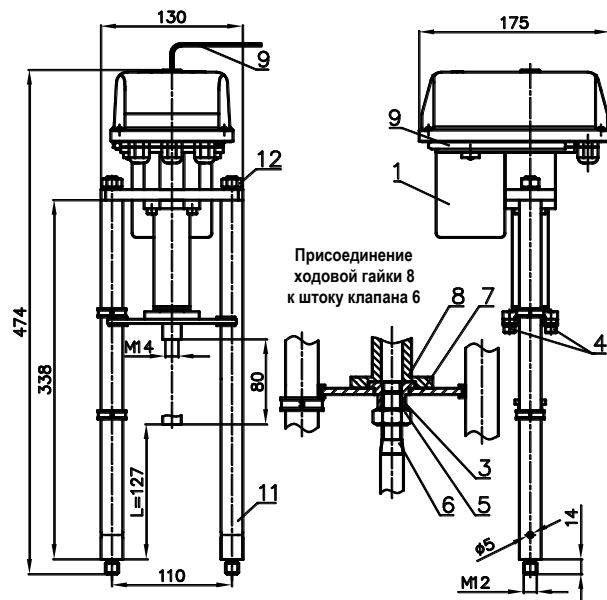
Рисунок 1 - ВЭП-131М
