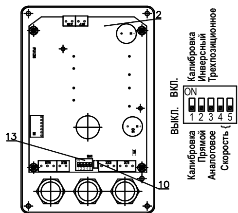
Рисунок 2. ВЭП-131М (вид при снятой крышке)
