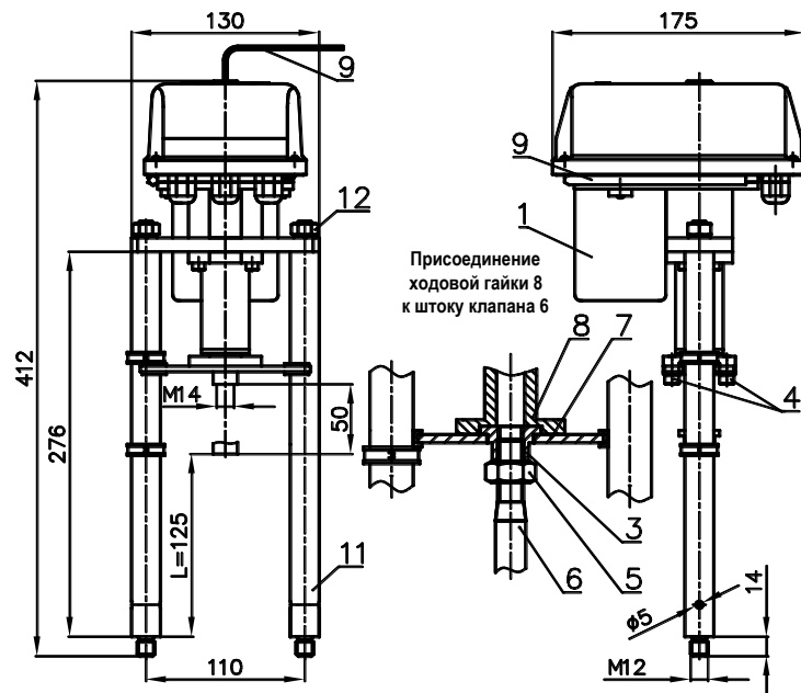
Рисунок 1 - ВЭП-131М
