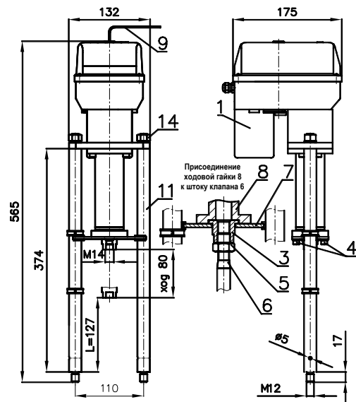
Рисунок 1 - ВЭП-135М
