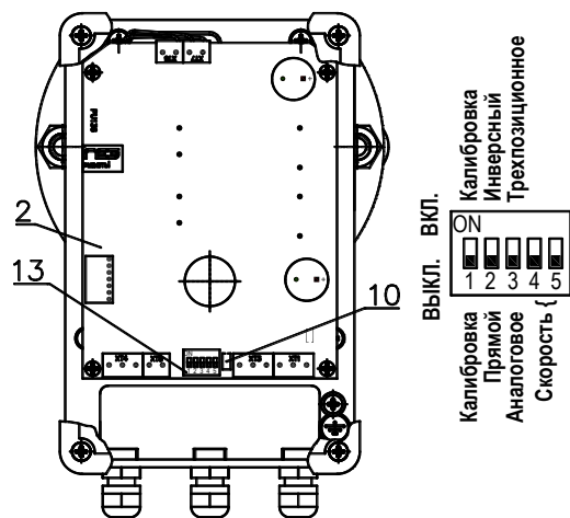
Рисунок 2. ВЭП-135М (вид при снятой крышке)
