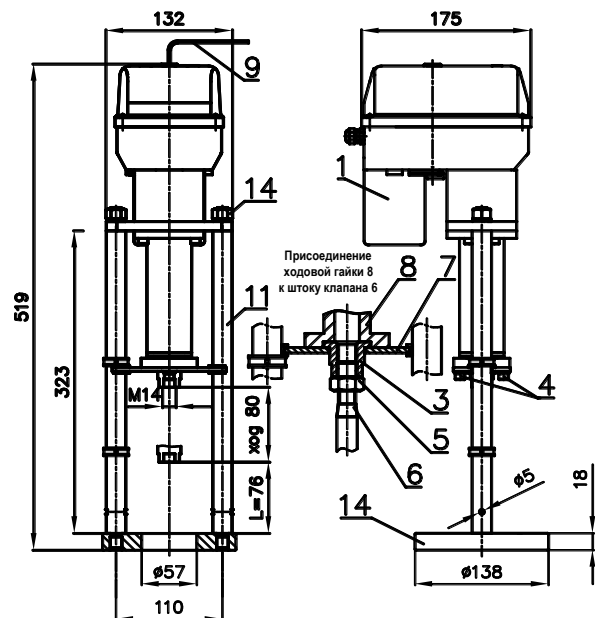
Рисунок 1 - ВЭП-138М
