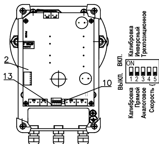
Рисунок 2. ВЭП-138М (вид при снятой крышке)
