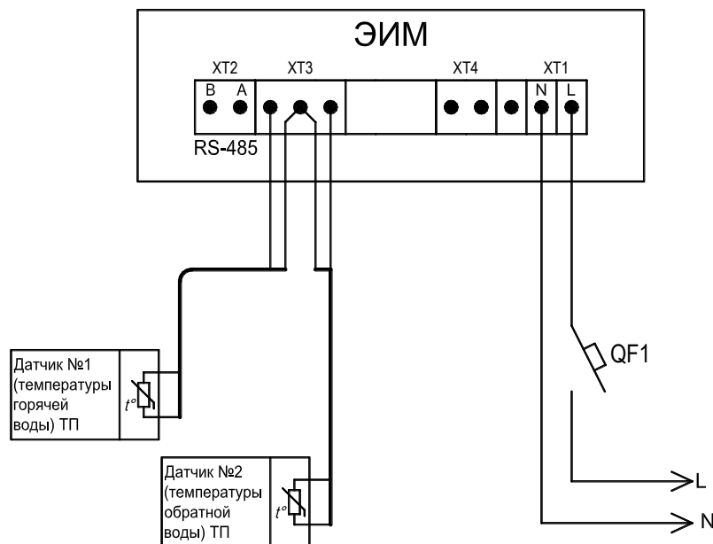
Рисунок 3 - Схема подключения в системе управления контуром ГВС (программа 20)
