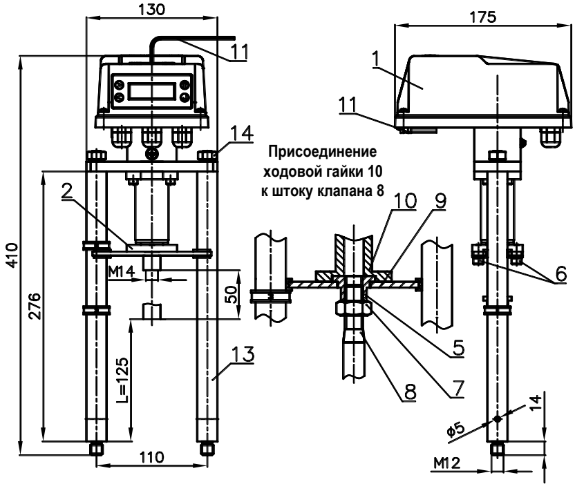
Рисунок 1 - ВЭП-225М
