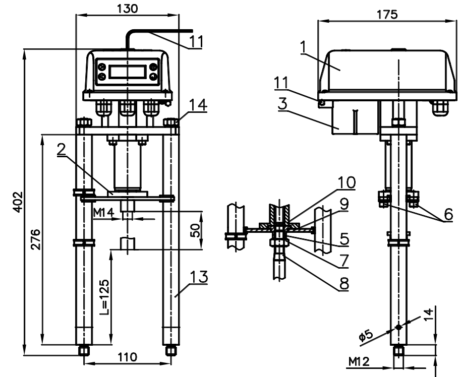
Рисунок 1 - ВЭП-245М
